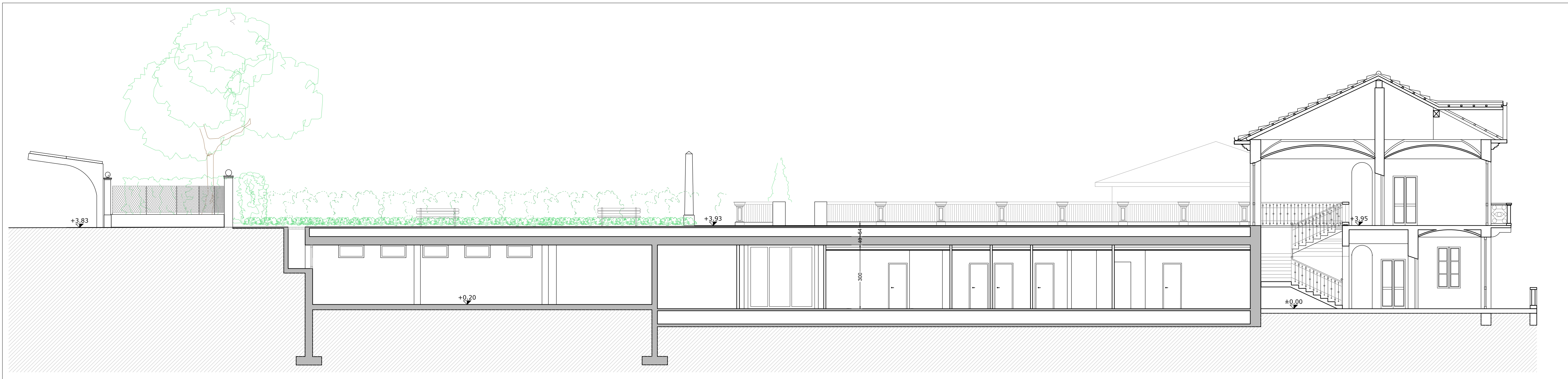
SEZIONE C-C
