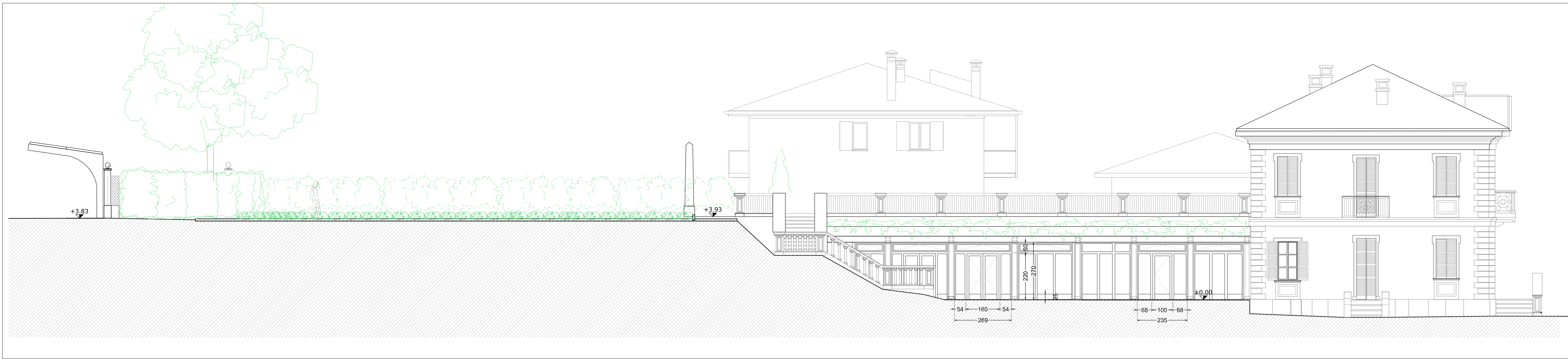
SEZIONE D-D
